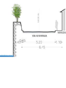
CORTE 40-40 CALLE CONFRATERNIDAD VÍA PAVIMENTADA 6.45 ml
