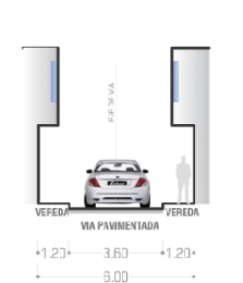
CORTE 32-32 CALLE MANANTIALES VÍA PAVIMENTADA 6.00
